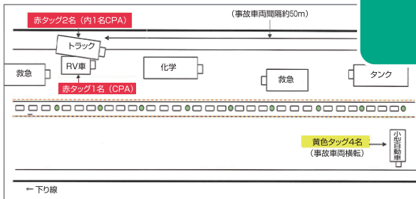
図2-1 現場概略図
